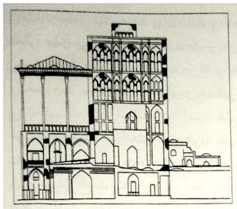
تصویر ۲- نقشه‌ای از نمای جنوبی کاخ عالی‌قاپو (محمدی‌اردکانی، ۱۳۸۶: ۵۴۰).
