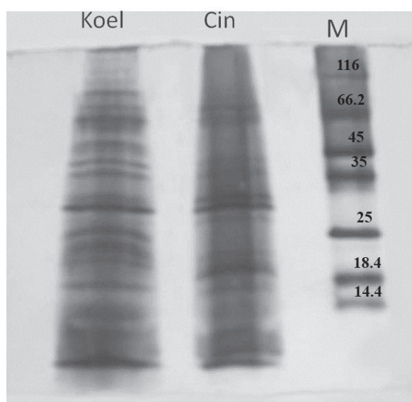
شکل ۲: تصویر الگوی بانندی بر روی ژل الکتروفورزی ۱۲٪ (رنگ آمیزی شده با نیترات نقره) (Koel: P. koelziana , Cin: P. cineraria , M: marker)
