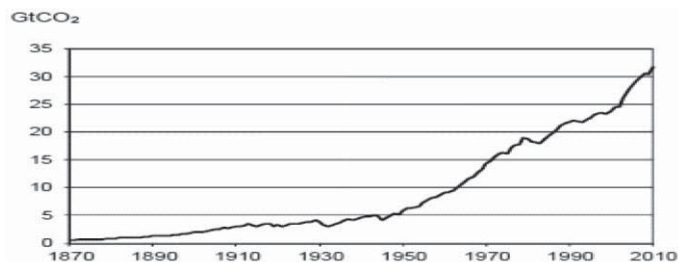
نمودار ۱. روند انتشار CO 2 در اثر احتراق سوخت‌های فسیلی
