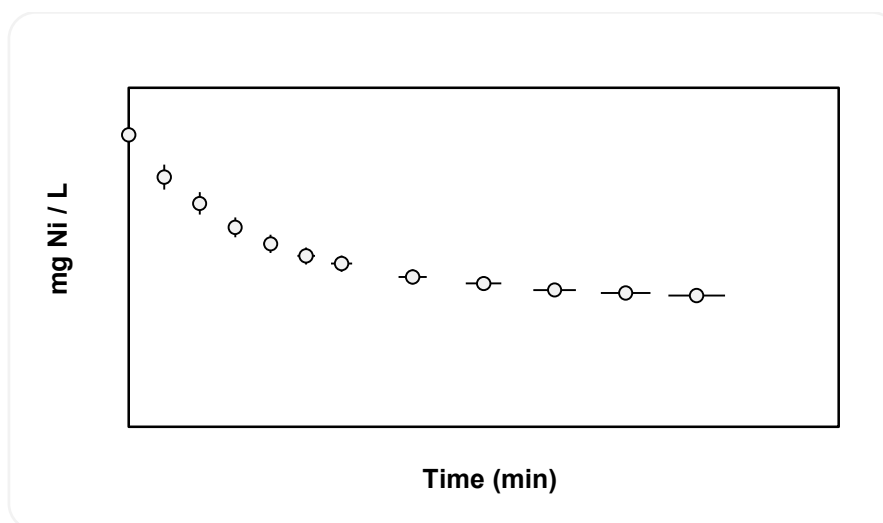
شکل شماره ۴: تأثیر افزایش غلظت فلز نیکل و زمان در جذب زیستی فلز نیکل به وسیله جلبک Gracilaria sp .
